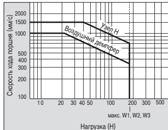
MY1H25 Горизонтальное столкновение; p=0.5 МПа
