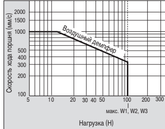
MY1H20 Горизонтальное столкновение; p=0.5 МПа
