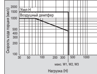
MY1H40 Горизонтальное столкновение; p=0.5 МПа
