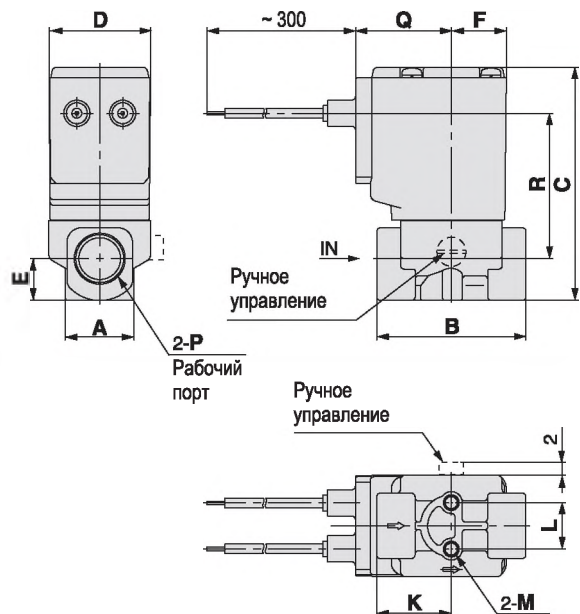
Залитый кабель. Тип G
