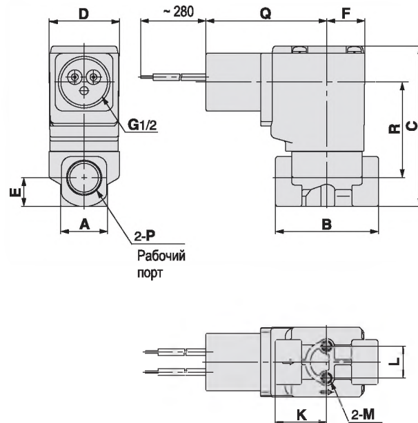
Кабелепровод. Тип С
